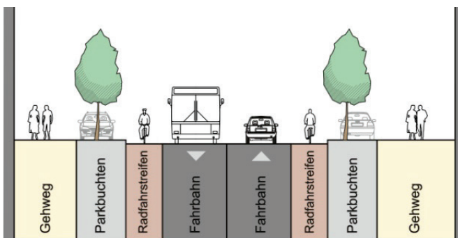
Planung für die Neuaufteilung des Straßenquerschnitts
