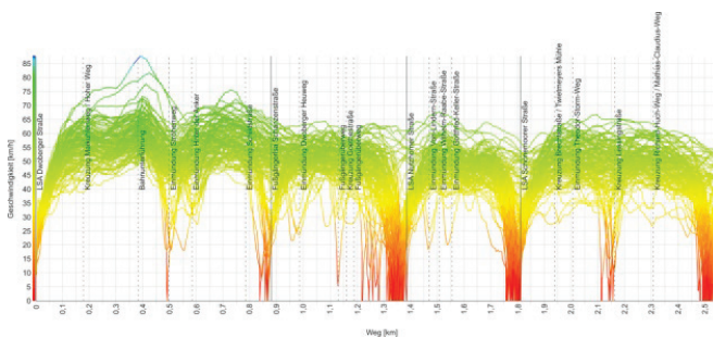
Weg-Geschwindigkeits-Diagramm Kfz
